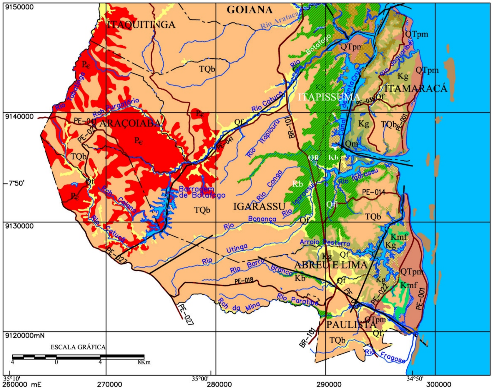
Figura 2.4 - MAPA GEOLÓGICO
